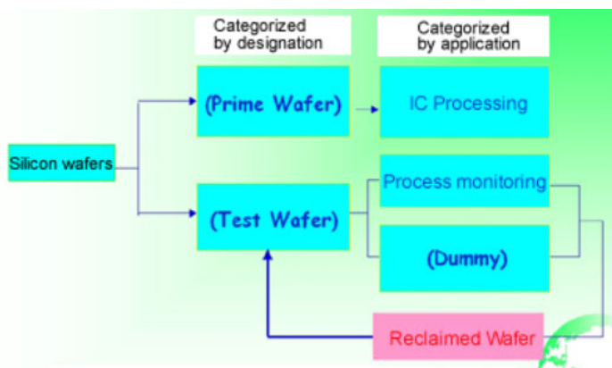
晶圓用途流程圖
